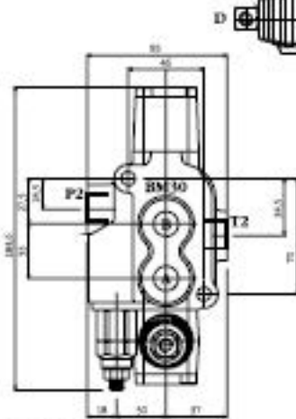
X = POSIZIONATORE - SPOOL CONTROL 2-3-12-14
