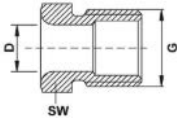
Raccord à bague à sertir pour monocône
