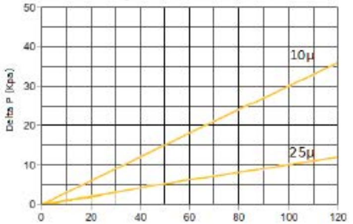
Pertes de charges des cartouches nominales
