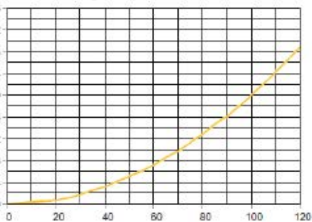
Pertes de charges corps du filtre EHFR100
