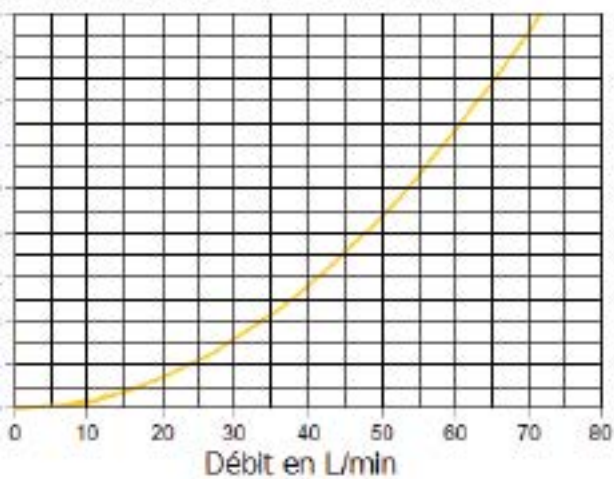
Pertes de charges corps du filtre EHFR160
