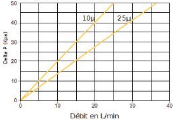
Pertes de charges des cartouches nominales
