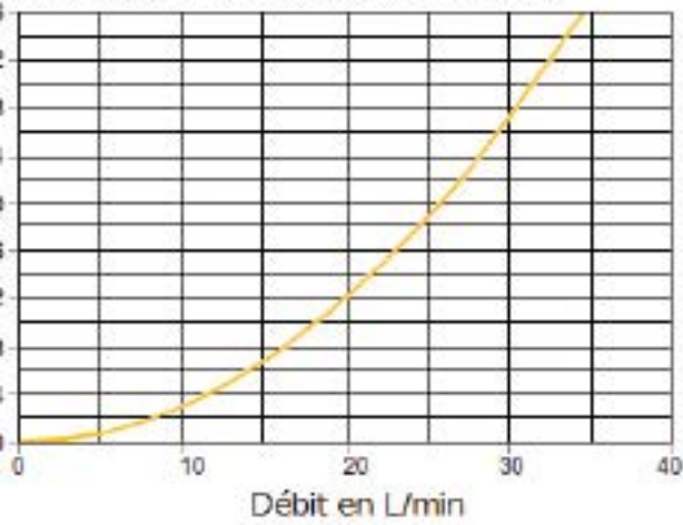
Pertes de charges corps du filtre EHFR130
